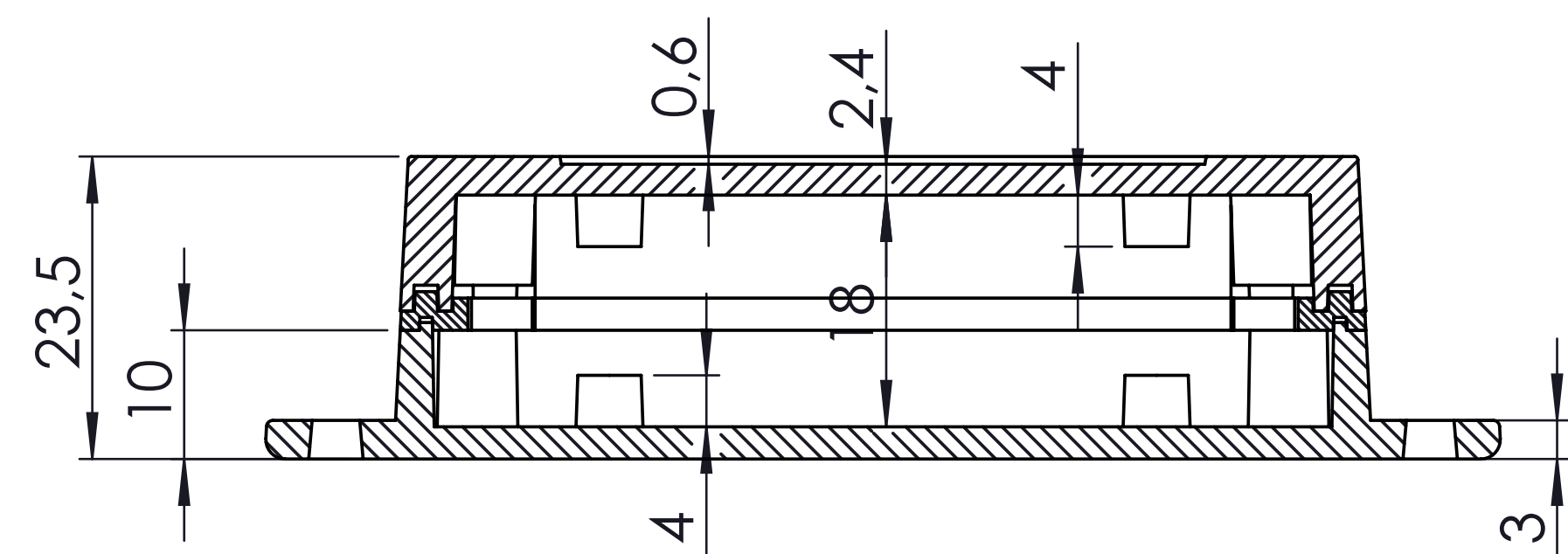
SECTION A-A
