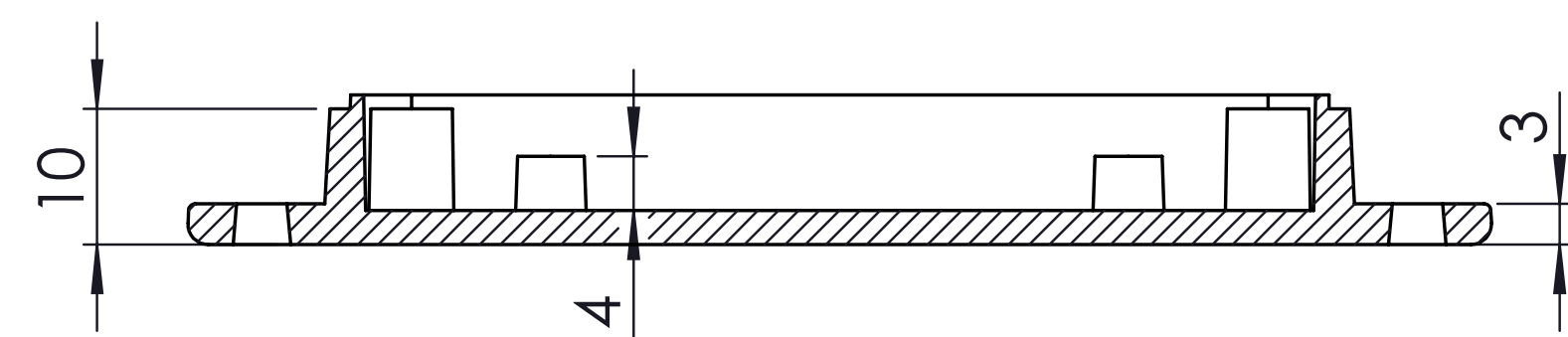
SECTION A-A
