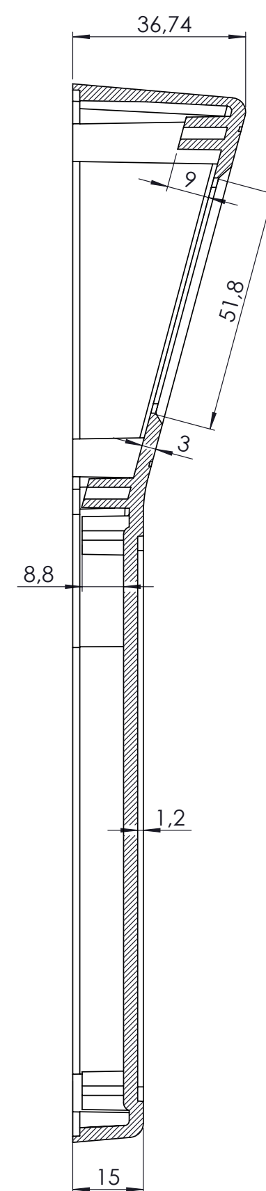
SECTION A-A
