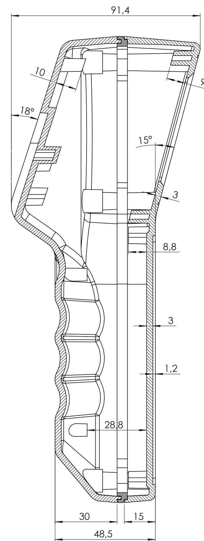
SECTION A-A
