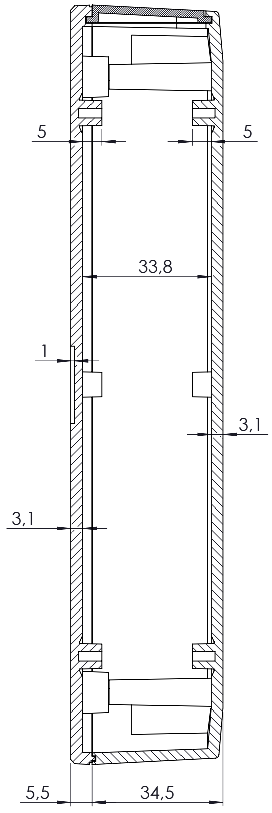
SECTION A-A
